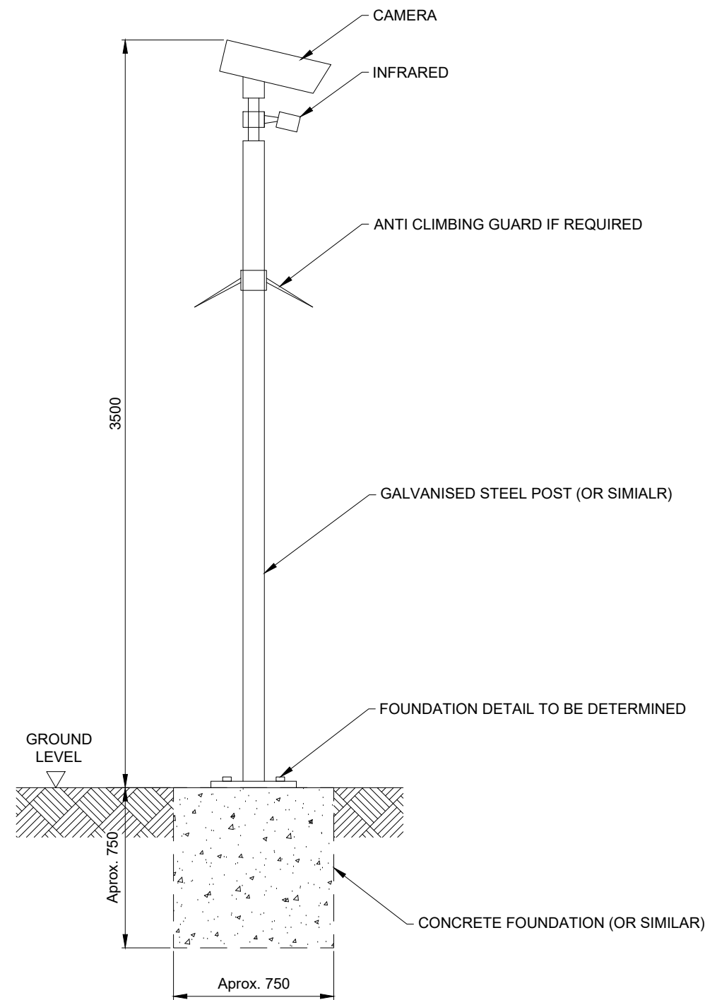
ELEVATION
